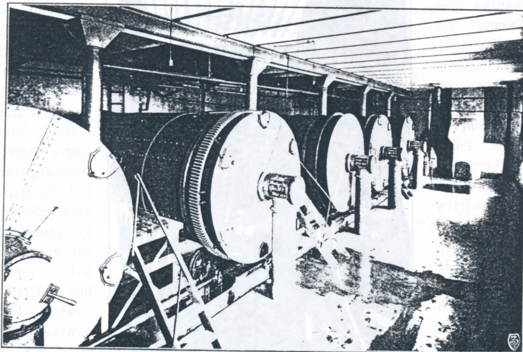
Trommelmölteri
