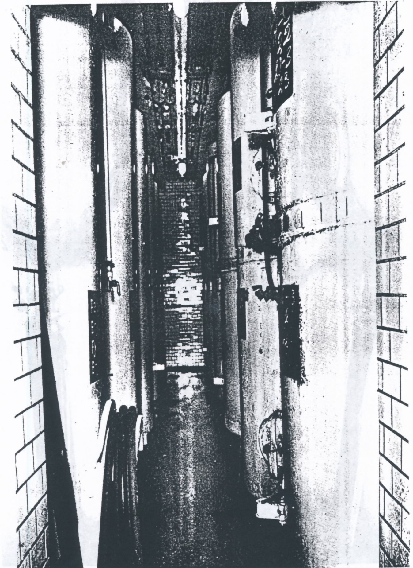
Lagerkällare No. I Glasmaljerade ståltanks, 1928
